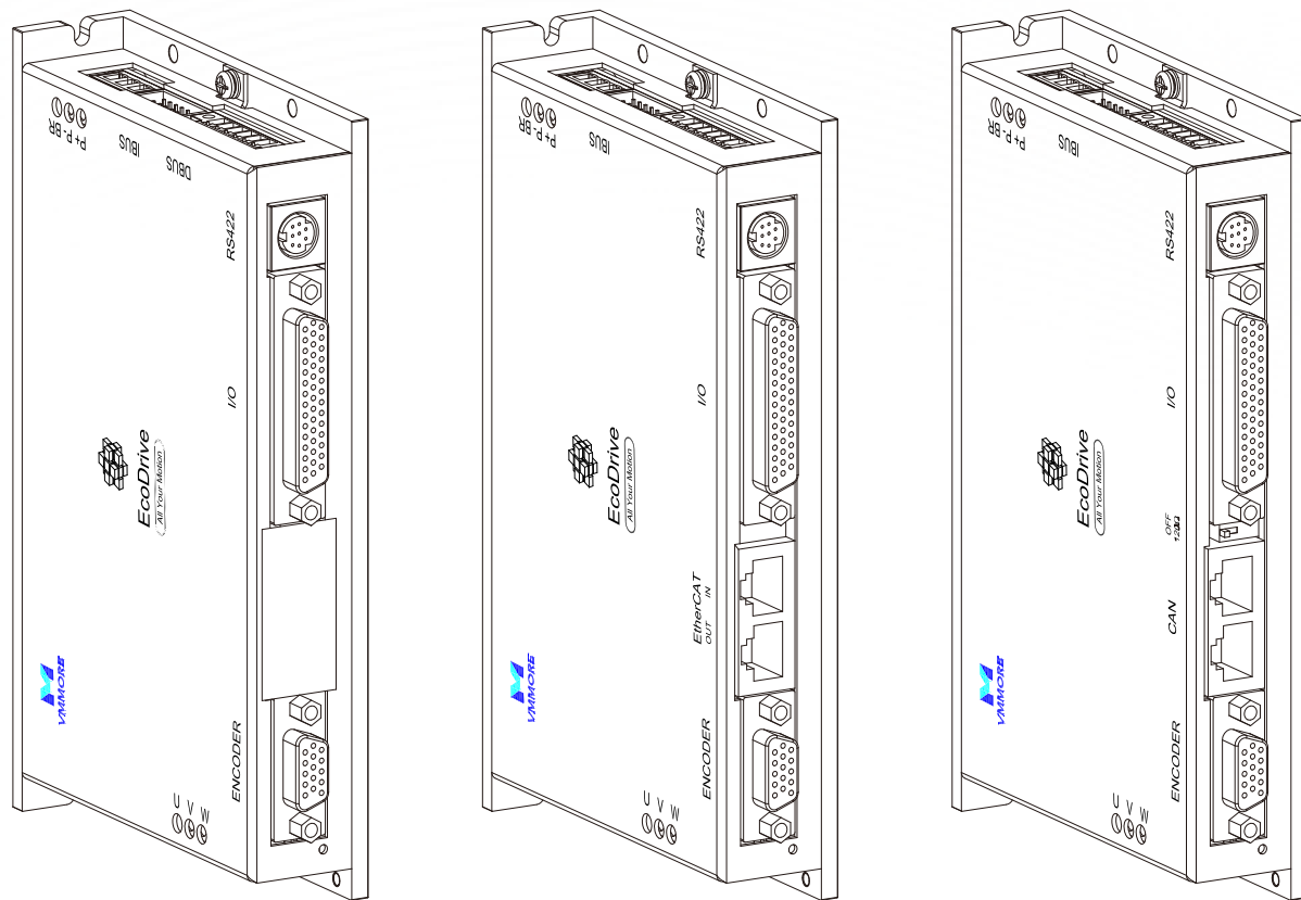
DBUS型驱动器
